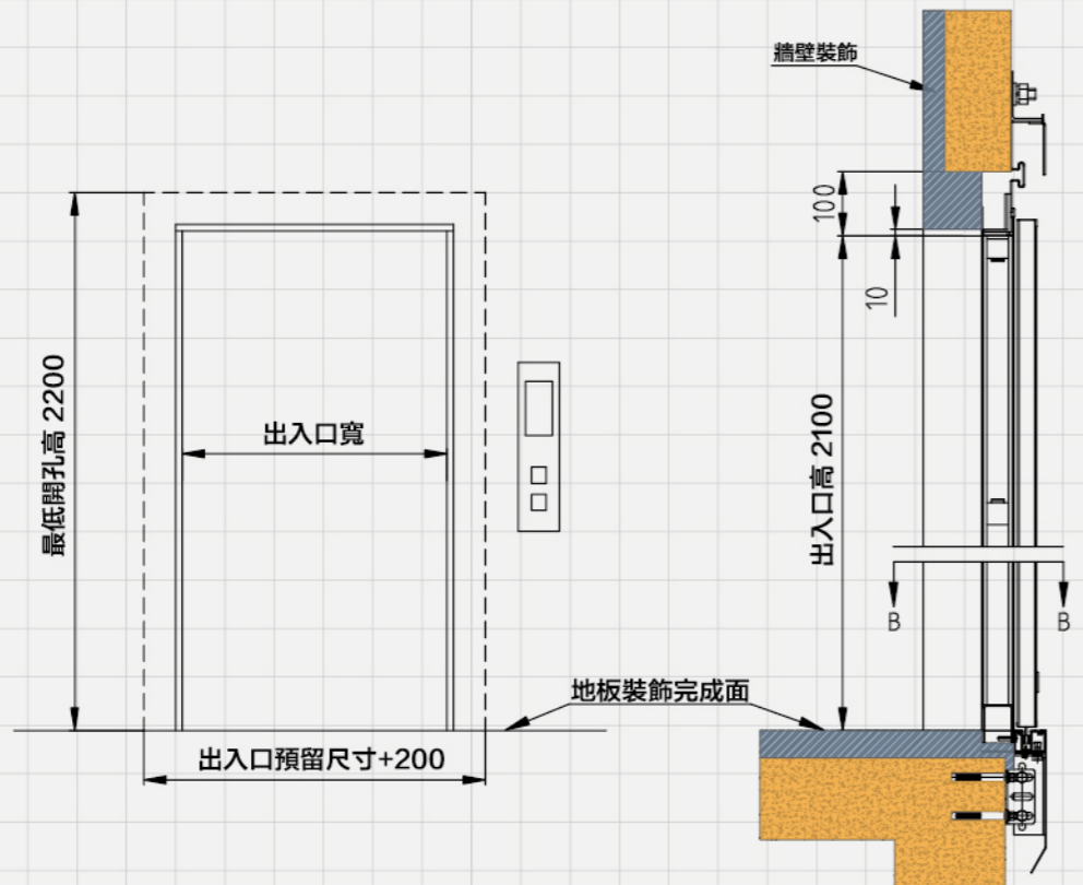
A-A斷面
