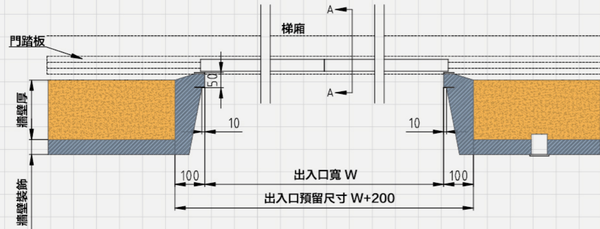
B-B斷面
