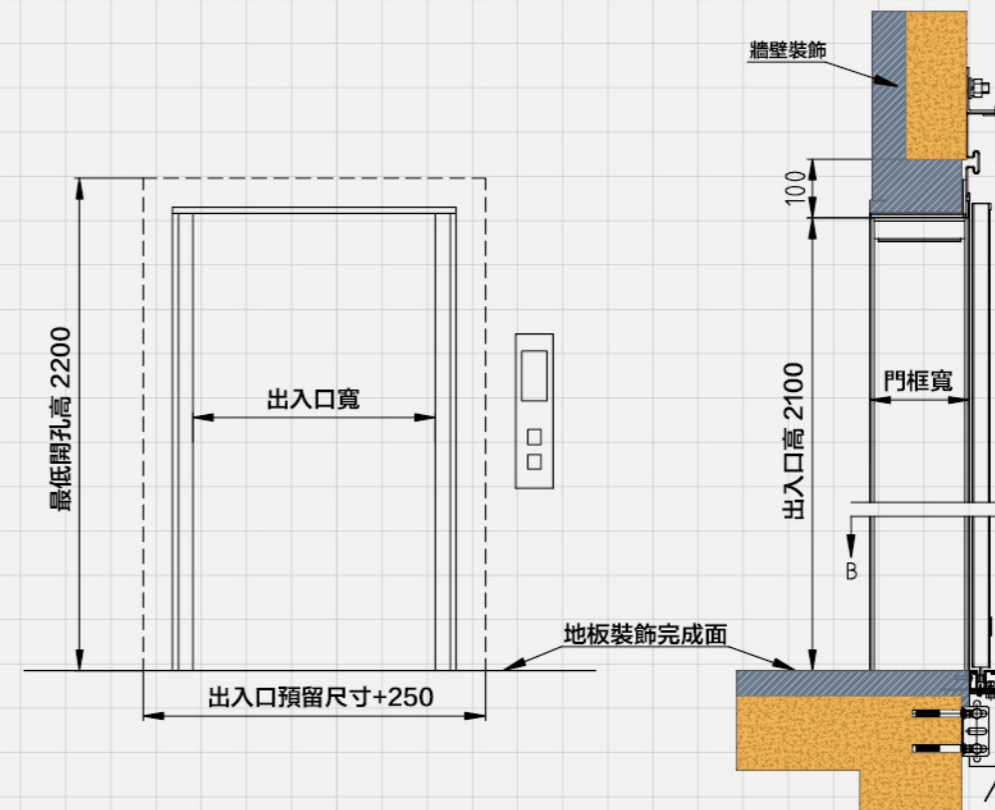
A-A斷面
