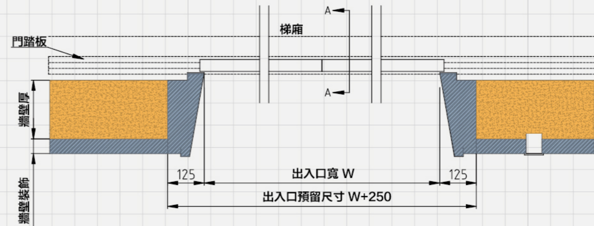
B-B斷面
